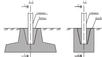
Рис. 2 Крепление щита знаков на опоре типа СКМ.
